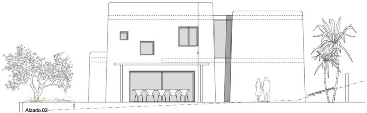
Alzado.02
