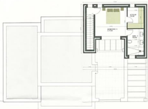
PLANTA PRIMERA ESCALA 1:50
