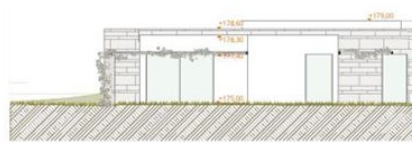
A-03.2 Alzado OESTE Hab. invitados 1:100
