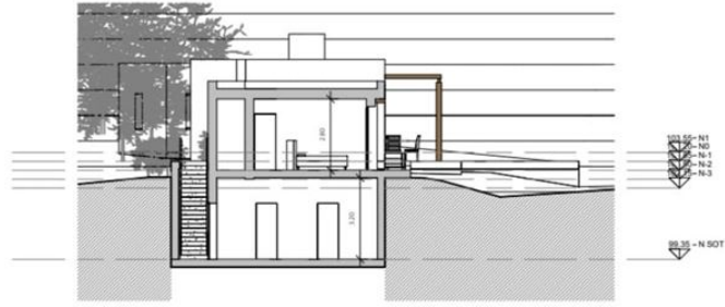
SECCIÓN 1
