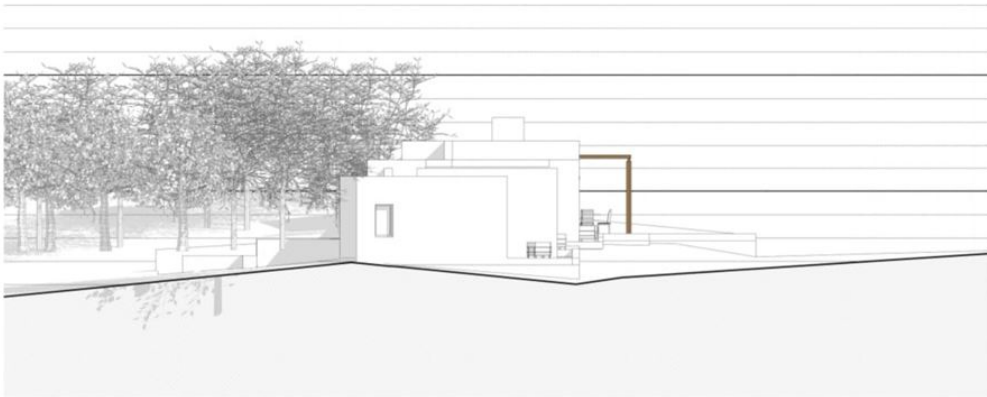
ALZADO OESTE
