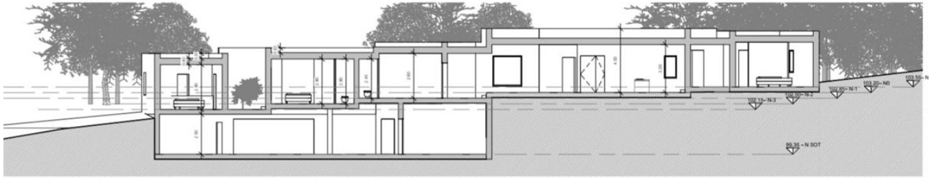
SECCIÓN 2
